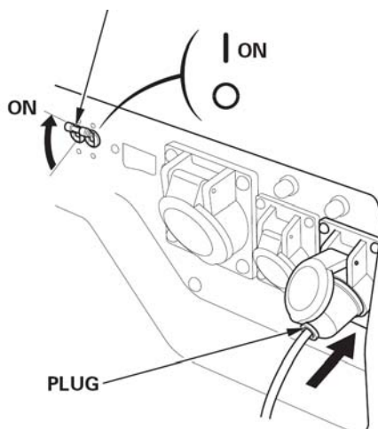
BEZPIECZNIK OBWODU PRĄDU ZMIENNEGO
