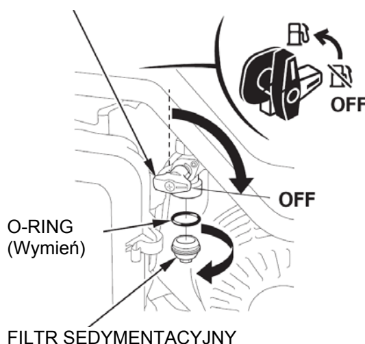
DŹWIGIENKA ZAWORU PALIWA
