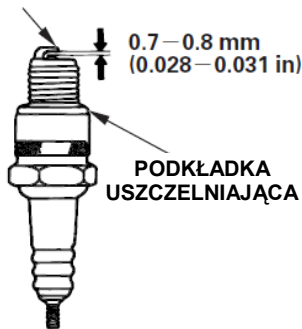
BOCZNA ELEKTRODA
