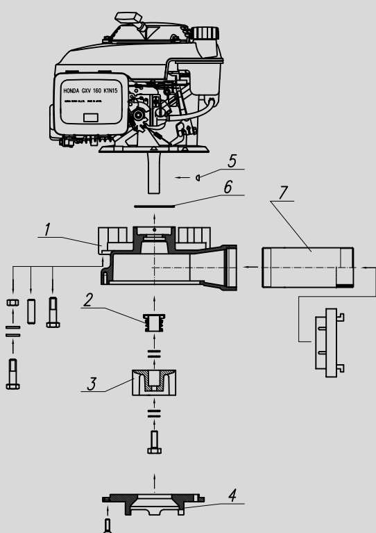
Rysunek techniczny
